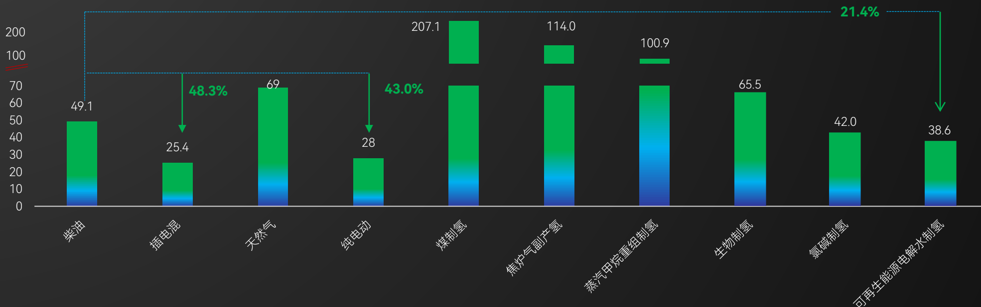
不同制氢工艺下全生命周期碳排放
