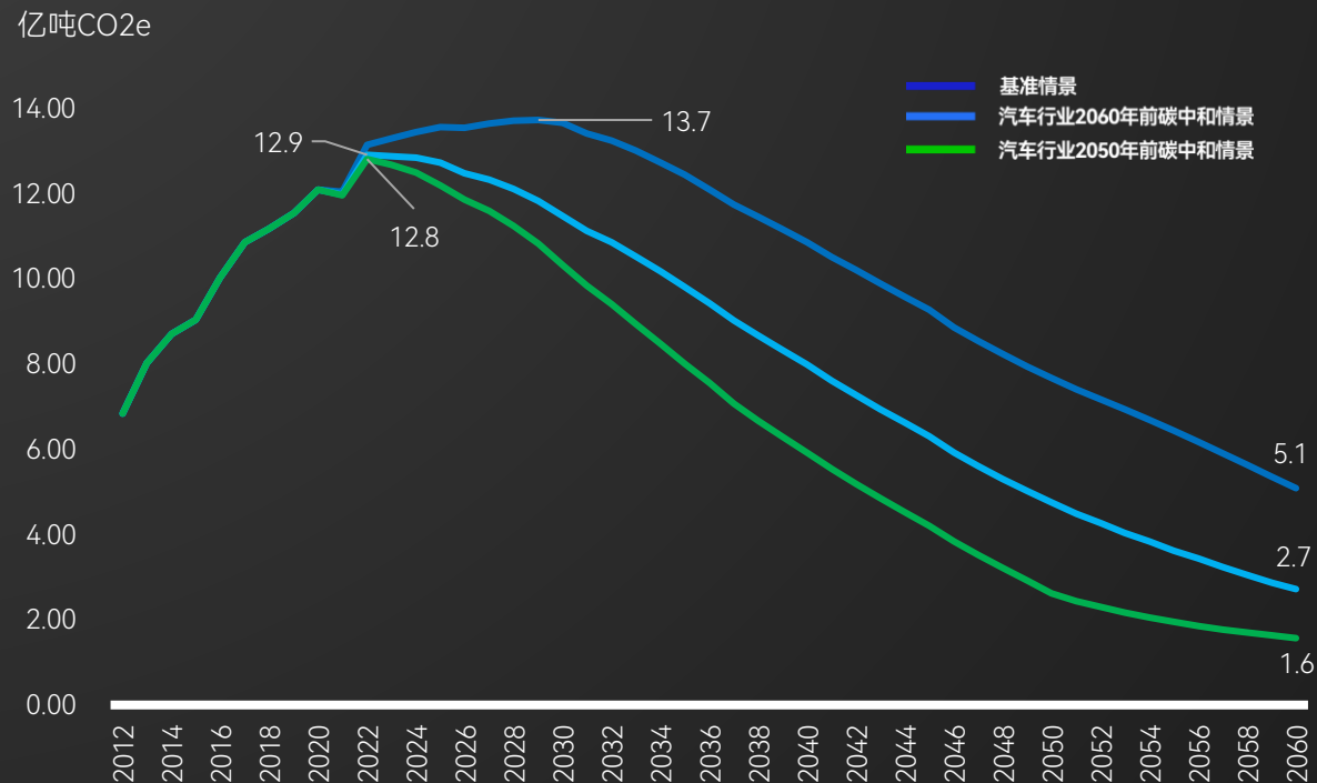
中国汽车车队生命周期碳排放预测
