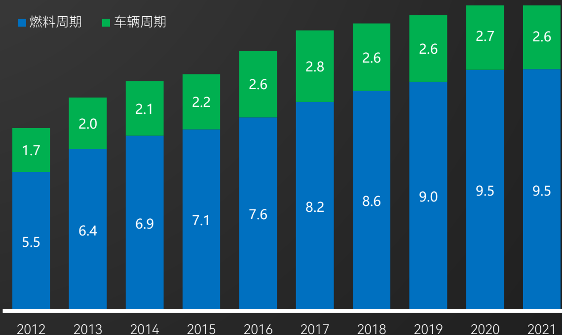
中国汽车车队生命周期碳排放
