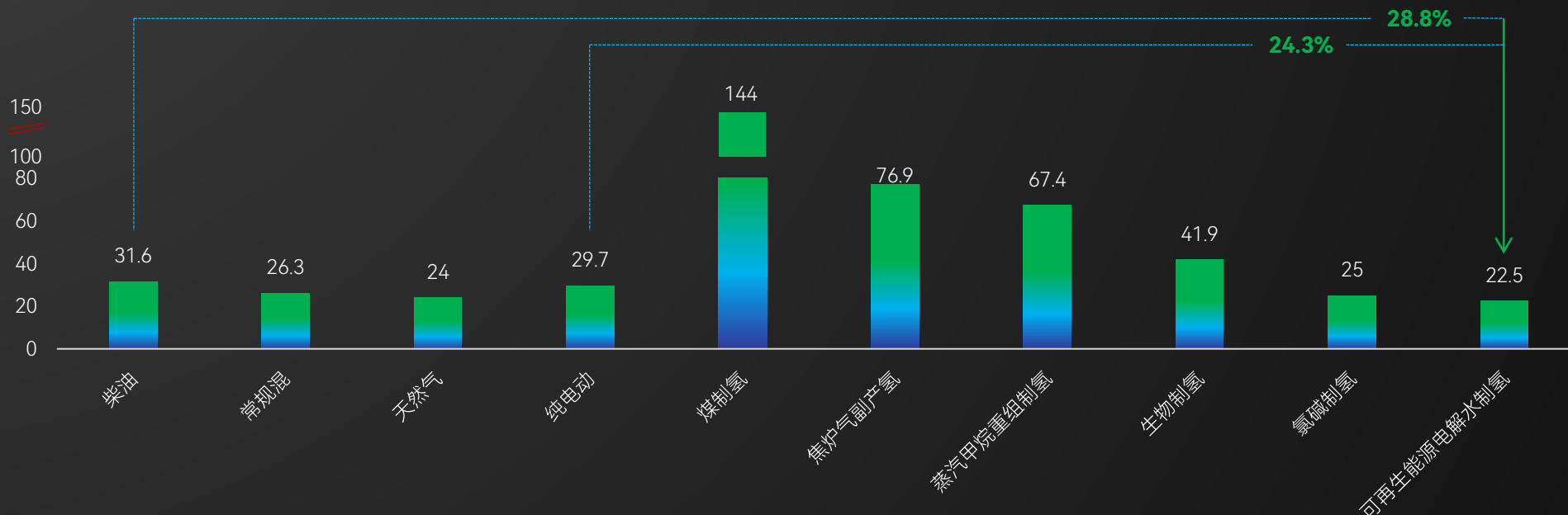
2021年不同燃料类型重型牵引车单位周转量的碳排放
